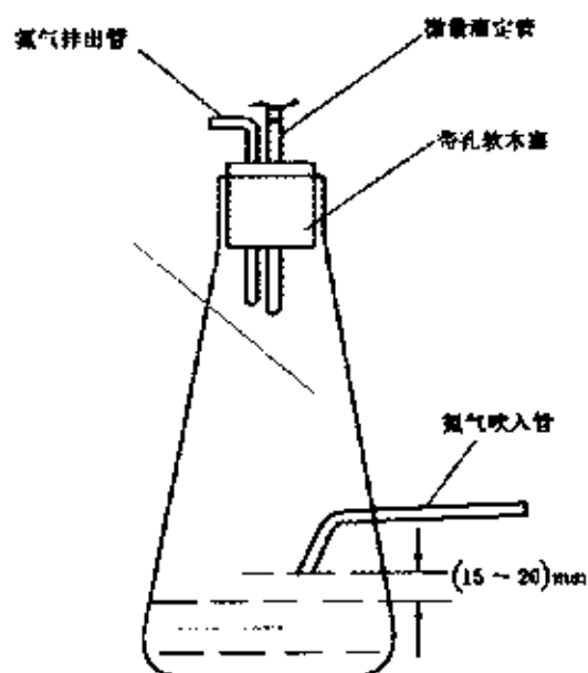
附图 1 带氮气吹管的具塞锥形瓶
