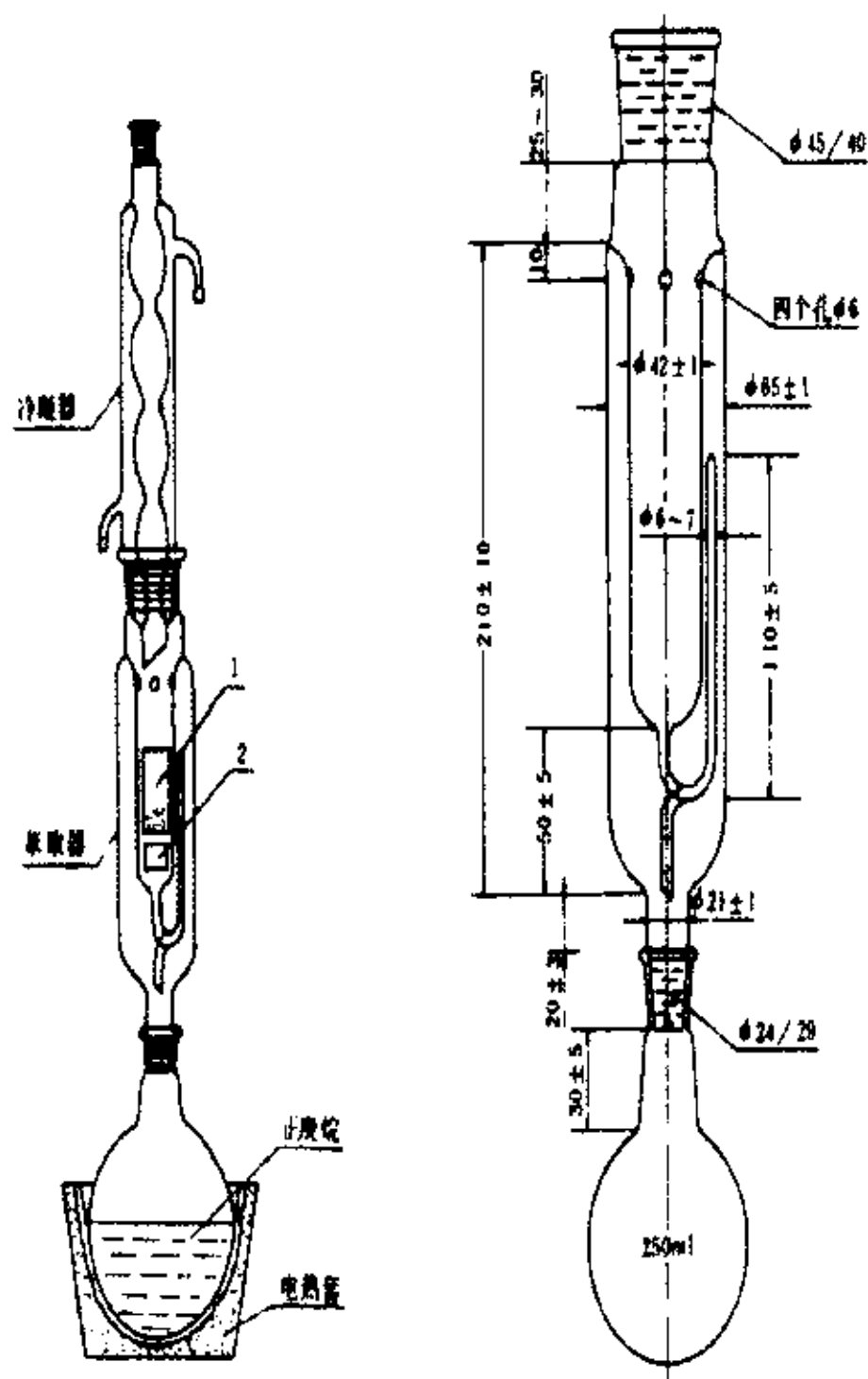
附图4 索氏萃取器（包括萃取装置和冷凝管）
