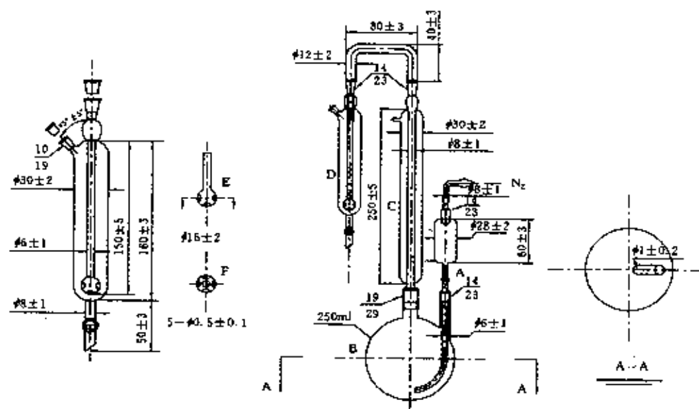
附图 2 酸化-吹气-吸收装置
